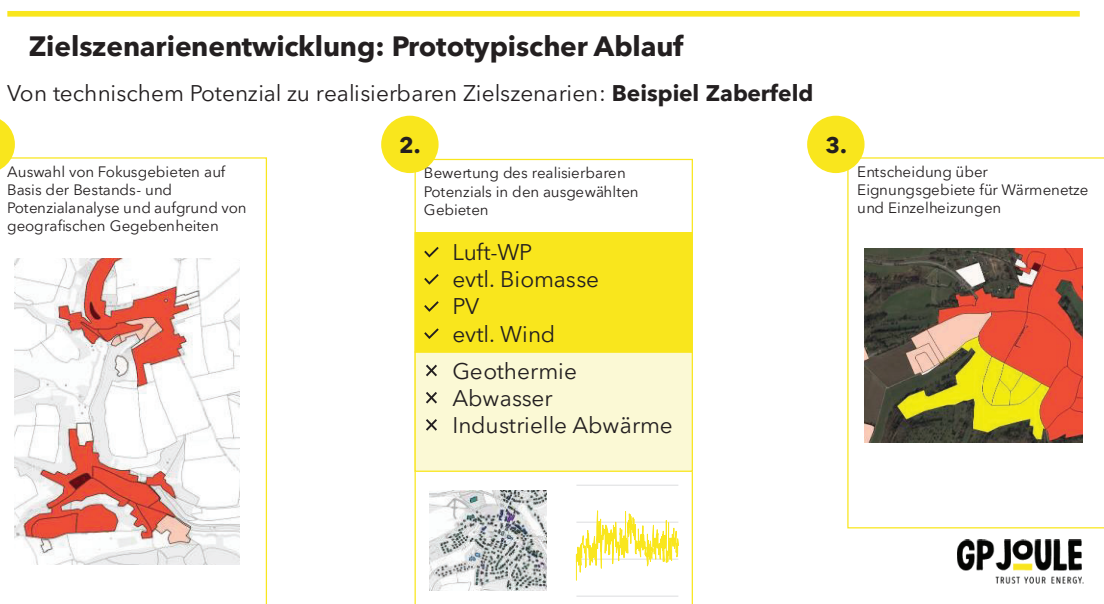
Abbildung 30: Prozessdarstellung Zielszenarienentwicklung
